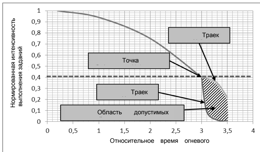
Рисунок 2 – Общий вид поведения функции показателя реализации возможностей в соответствии с подходами теории бифуркаций.
