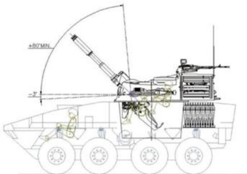
Рисунок 1 – Вариант 82-мм самоходного миномета «Василек-С» на колесном шасси типа БТР (БРДМ)
