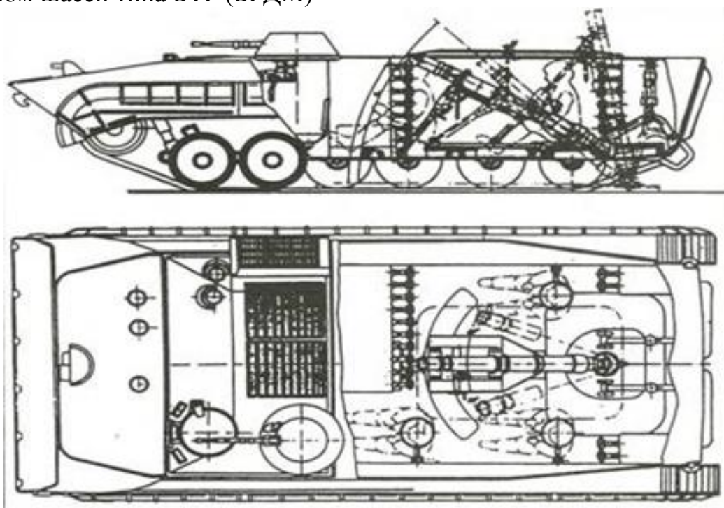
Рисунок 2 – 120-мм самоходный миномет на шасси типа БМП-1, МТЛБ (вариант без башни, с раздвижными люками)
