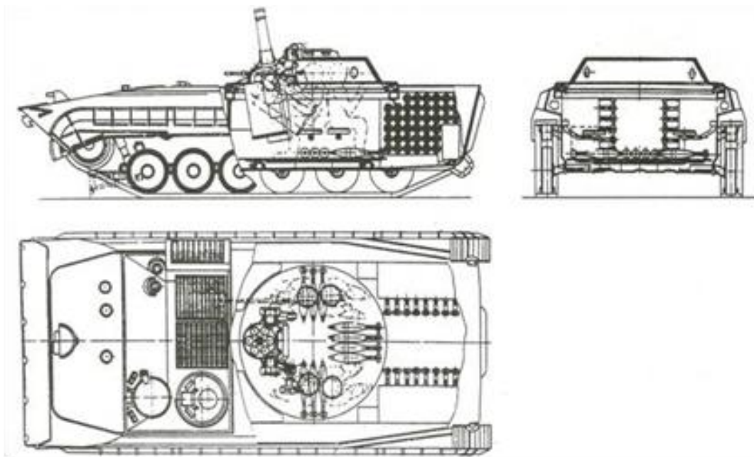
Рисунок 3 – 120мм самоходный миномет на базе БМП-1
